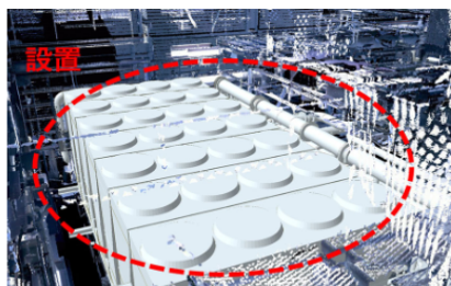
点群データ+BIMによる撤去後の画像
